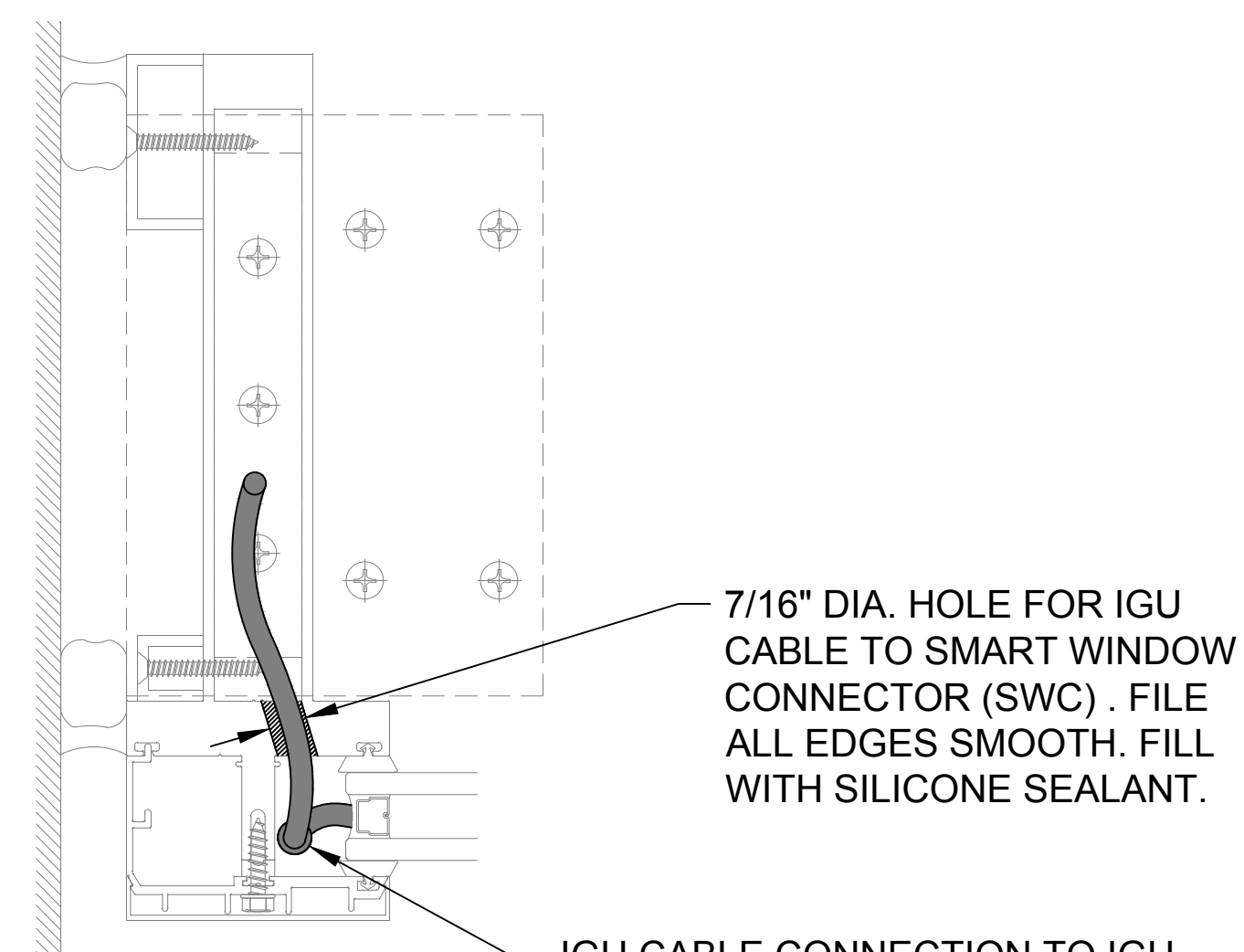
DETAIL 5 LEFT JAMB
